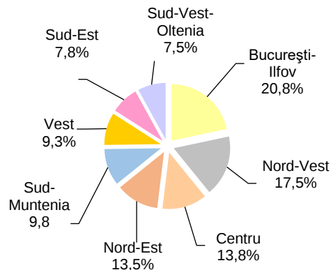
Graficul nr. 2 Înmatriculări noi de vehicule rutiere pentru transportul mărfurilor în perioada 1.I - 30.IX 2022
