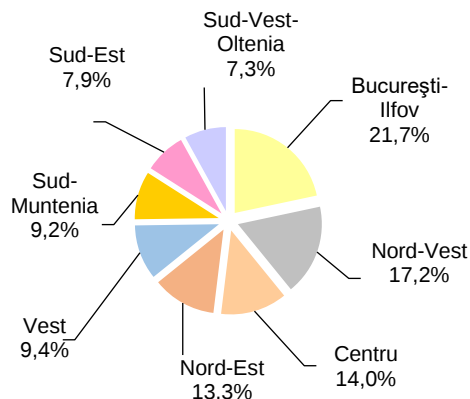
Graficul nr.4 Înmatriculări noi de vehicule rutiere pentru transportul mărfurilor în trimestrul III 2022
