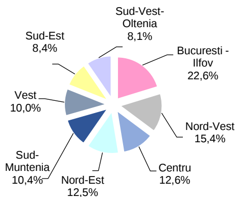
Graficul nr. 1 Înmatriculări noi de vehicule rutiere pentru transportul pasagerilor în perioada 1.I - 30.IX 2022
