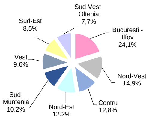
Graficul nr.3 Înmatriculări noi de vehicule rutiere pentru transportul pasagerilor în trimestrul III 2022
