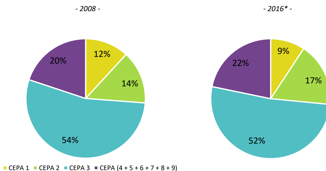
Graficul 4.8. Structura producției totale de servicii de protecția mediului pe principalele domenii de mediu CEPA în anii 2008 și 2016
