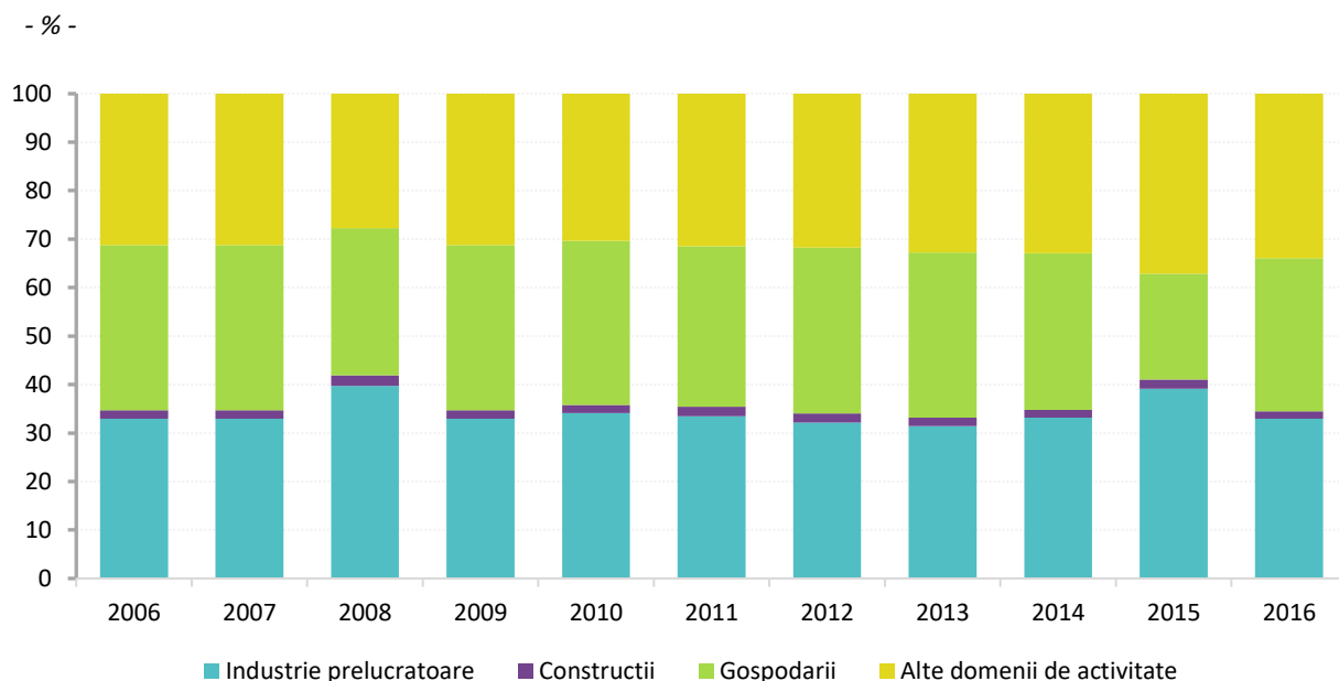
Graficul 5.10. Distribuția taxelor pe poluare pe domenii de activitate în perioada 2006 – 2016
