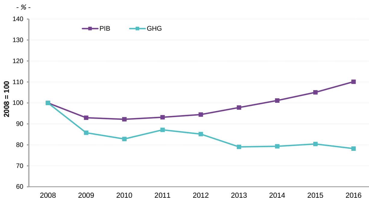
Graficul 2.5. Evoluția emisiilor de gaze cu efect de seră și a PIB, în perioada 2008-2016
