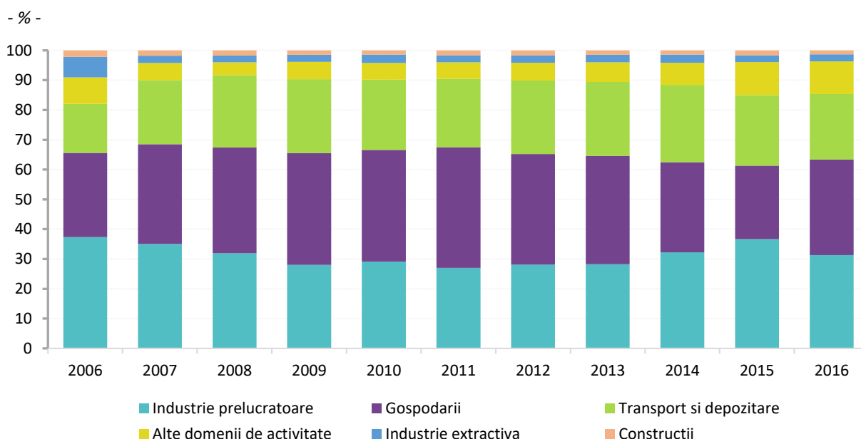
Graficul 5.12. Distribuția taxelor de mediu pe domenii de activitate în perioada 2006 – 2016
