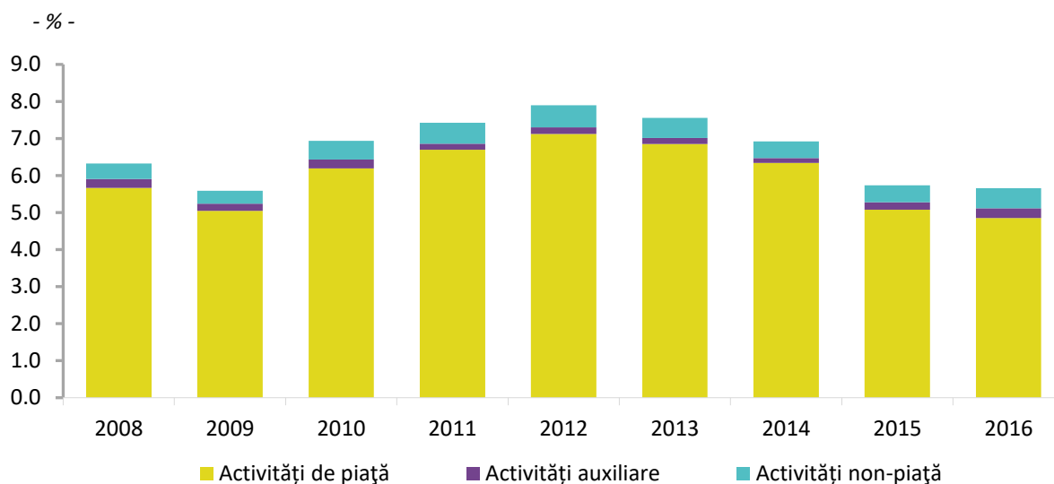
Graficul 3.4. Ponderea în PIB a valorii producției de bunuri și servicii de mediu, pe activități de piață, non – piață și auxiliare, în perioada 2008 – 2016
