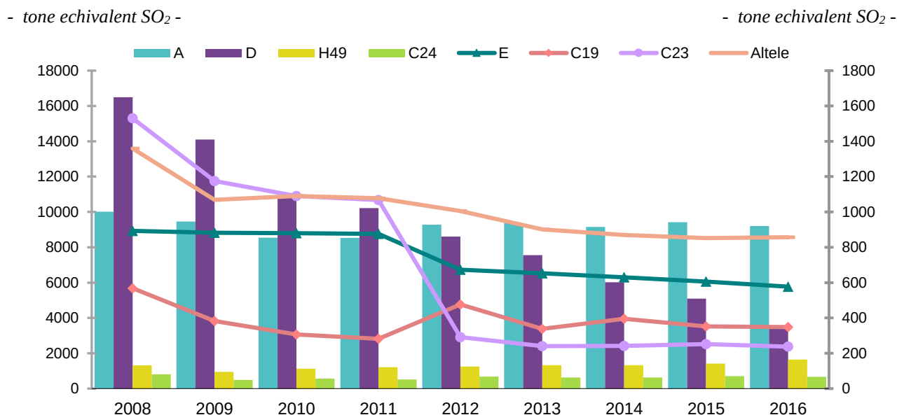
Graficul 2.8. Evoluția emisiilor de gaze acidifiante pe principalele activități economice în perioada 2008 – 2016
