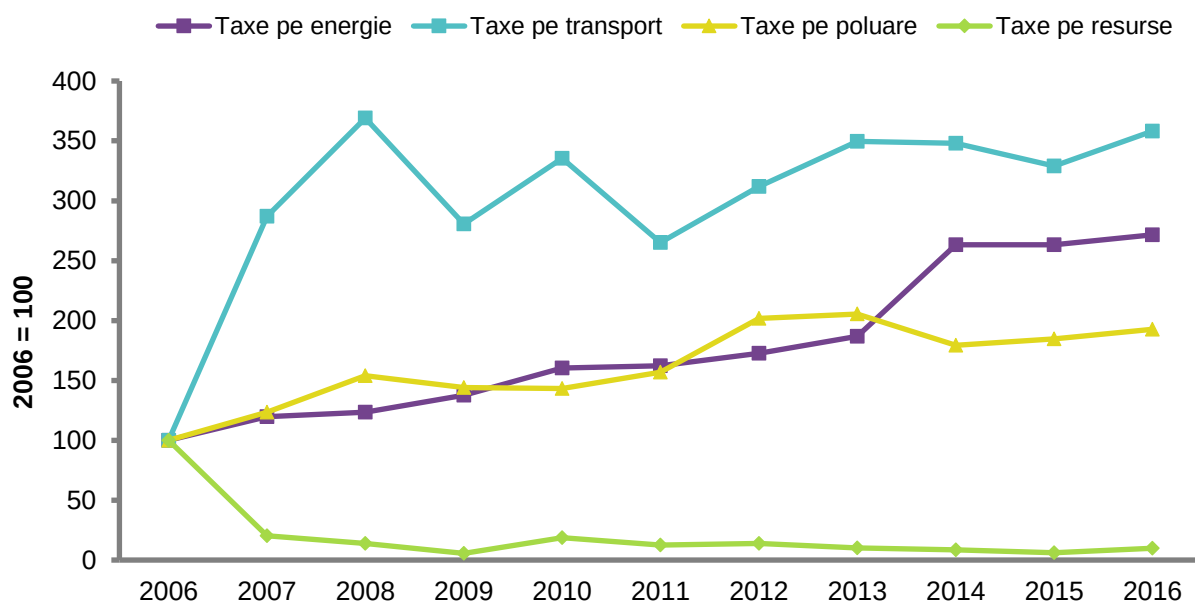
Graficul 5.4. Variația taxelor de mediu, pe categorii de taxe în perioada 2006 – 2016
