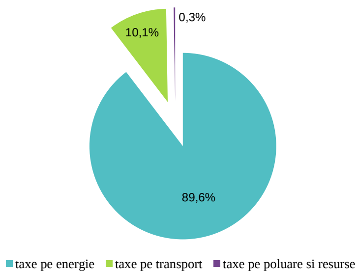
Graficul 5.5. Structura taxelor de mediu pe categorii de taxe în anul 2016
