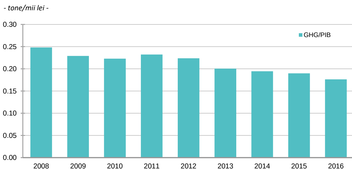
Graficul 2.6. Evoluția intensității emisiilor de gaze cu efect de seră, în perioada 2008-2016
