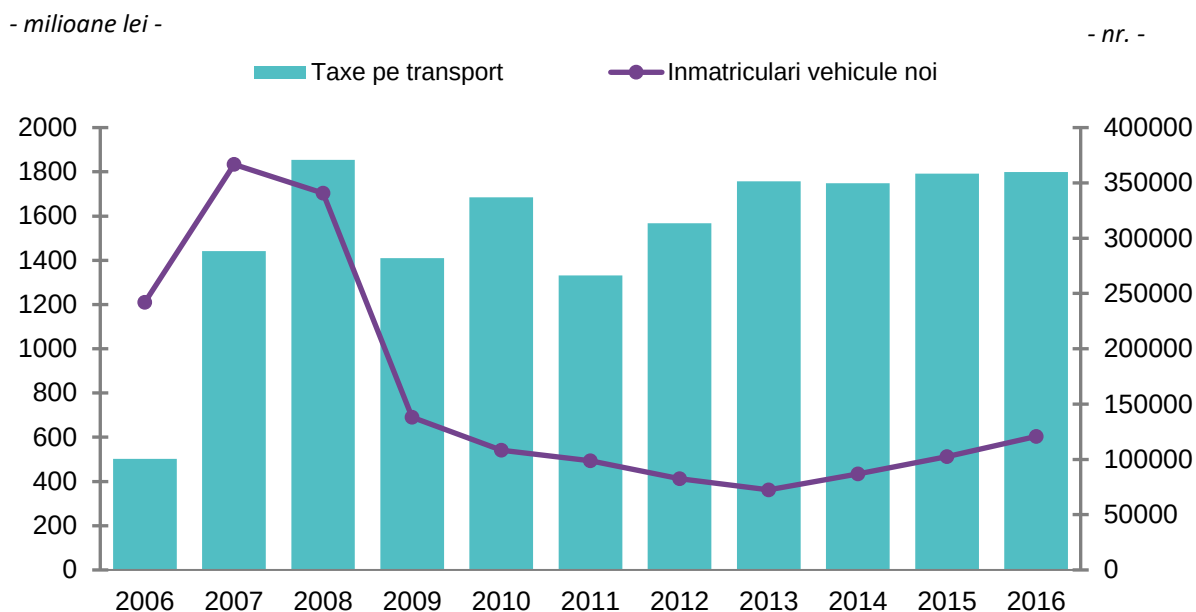
Graficul 5.7. Variația taxelor pe transport și a numărului de înmatriculări de autovehicule noi în perioada 2006 – 2016
