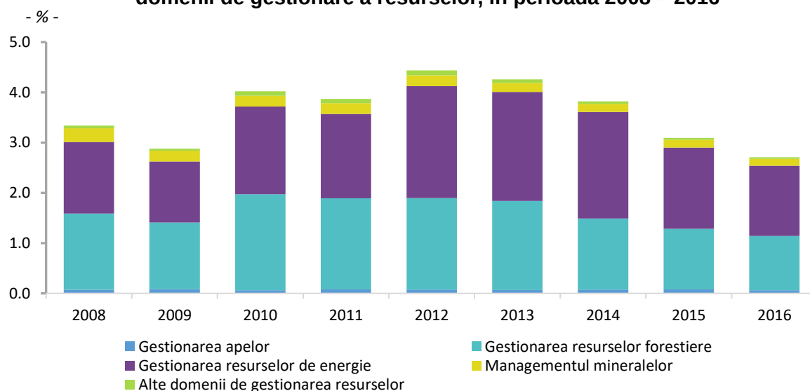
Graficul 3.3. Ponderea în PIB a valorii producției de bunuri și servicii de mediu, pe domenii de gestionare a resurselor, în perioada 2008 – 2016
