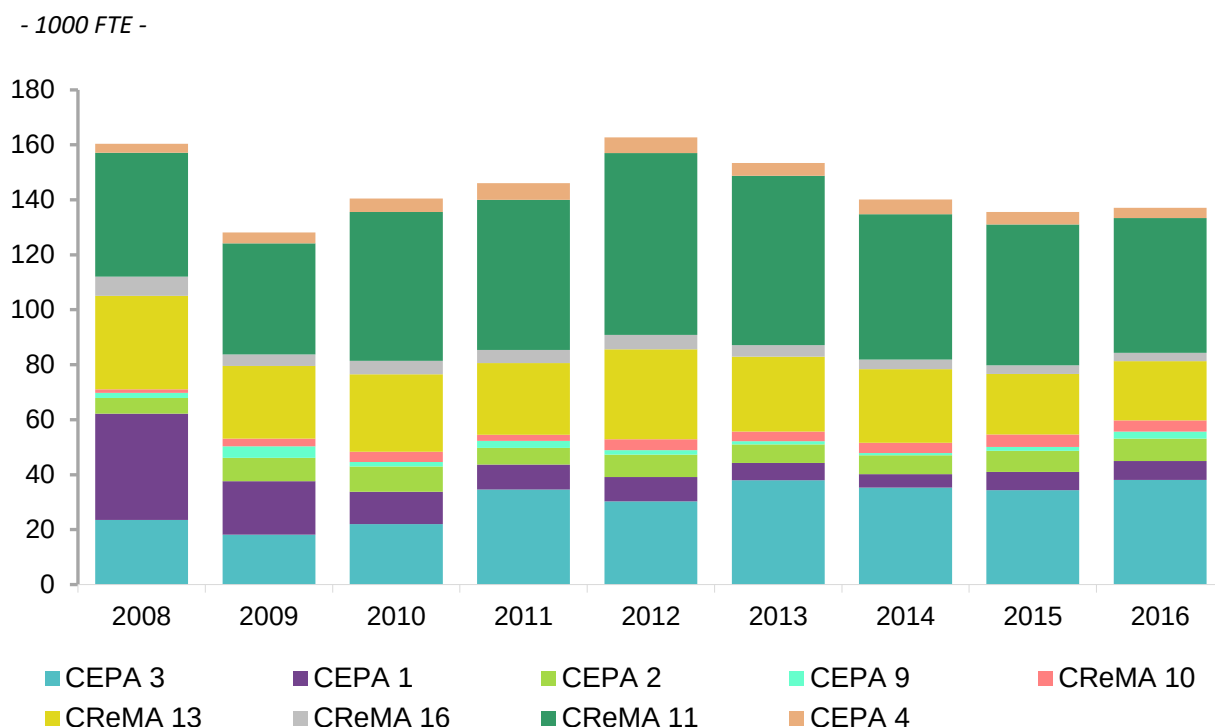
Graficul 3.10. Populația ocupată din EGSS pe principalele domenii de mediu în perioada 2008 – 2016
