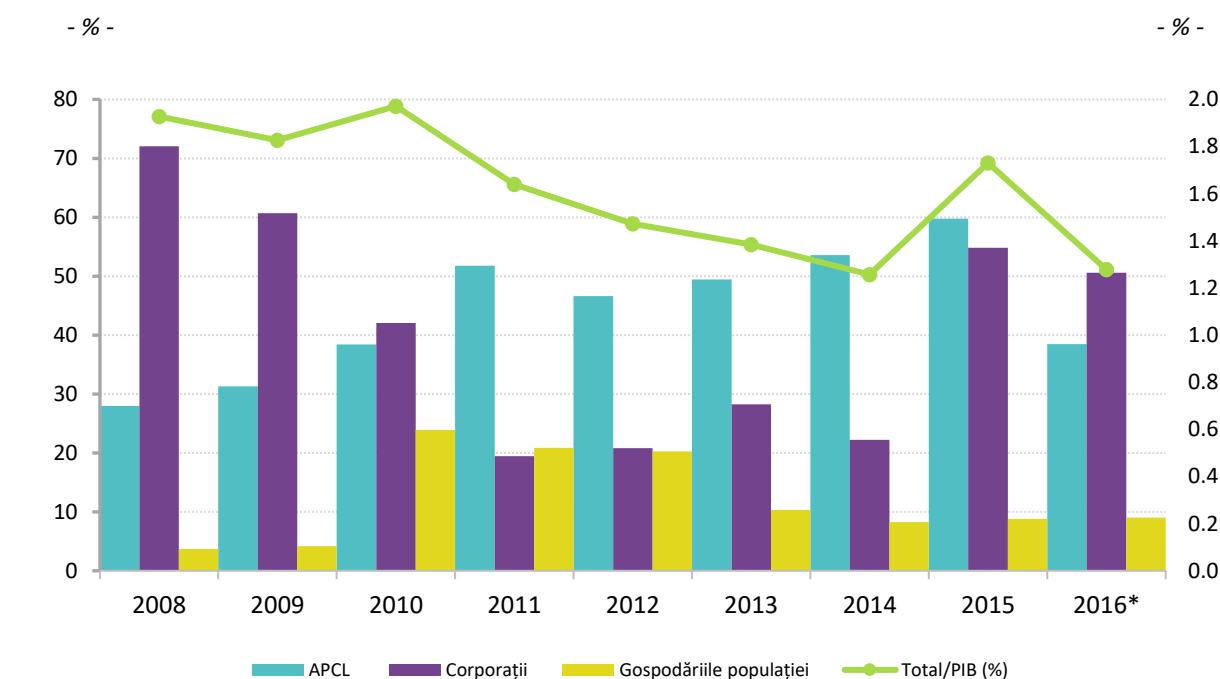
Graficul 4.1. Structura cheltuielilor naționale de protecția mediului pe sectoare instituționale și ponderea cheltuielilor naționale totale în PIB în perioada 2008-2016
