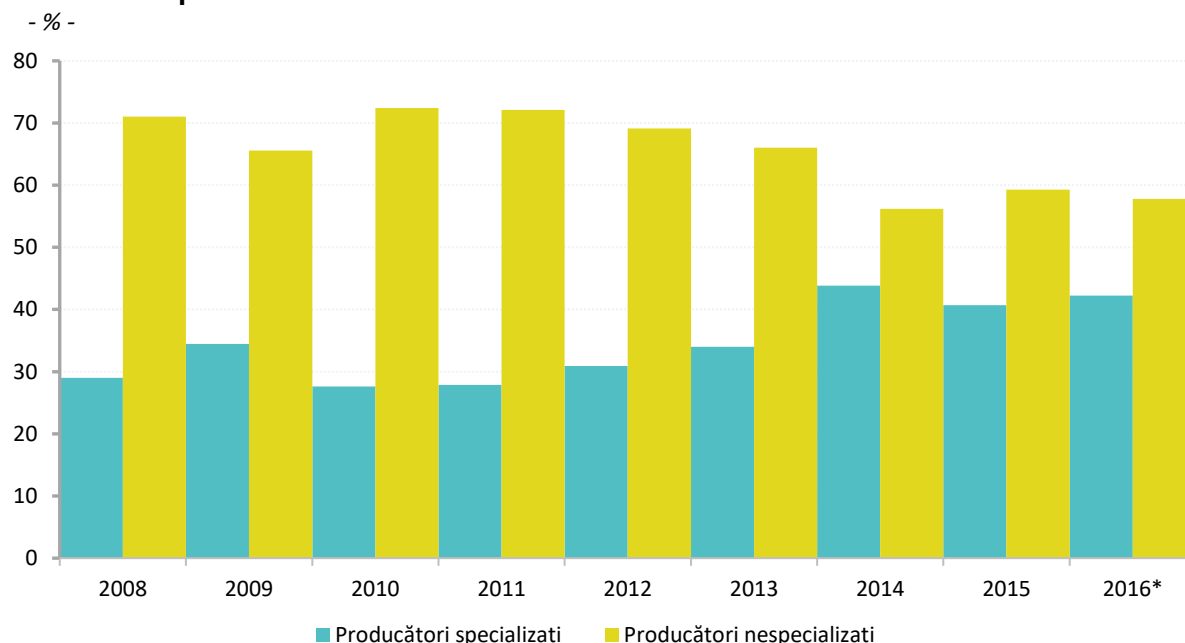
Graficul 4.2. Structura consumului intermediar pe categorii de producători în perioada 2008-2016
