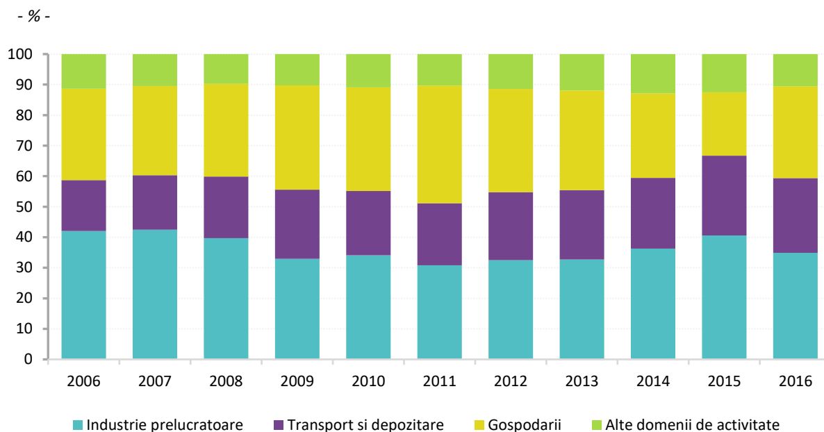
Graficul 5.8. Distribuția taxelor pe energie pe principalele domenii de activitate în perioada 2006 – 2016
