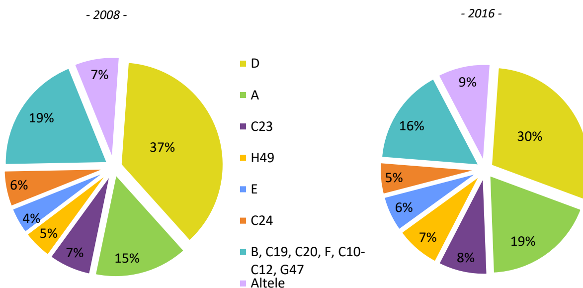
Graficul 2.4. Structura emisiilor de gaze cu efect de seră pe principalele activități economice în anii 2008 și 2016
