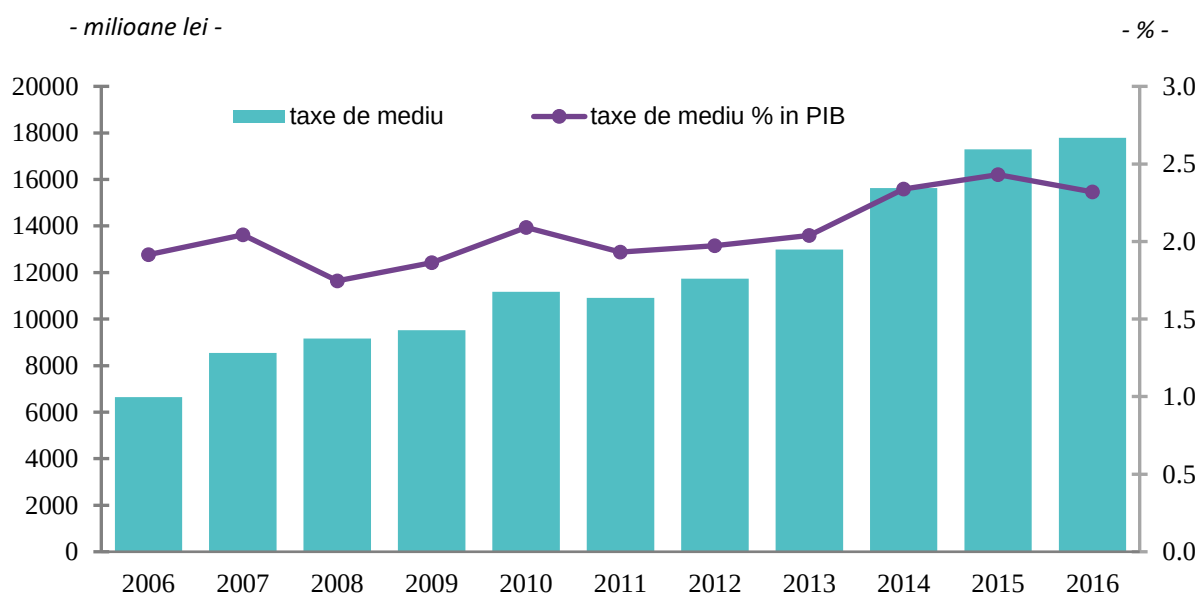
Graficul 5.1. Taxele de mediu și ponderea acestora în PIB în perioada 2006 – 2016
