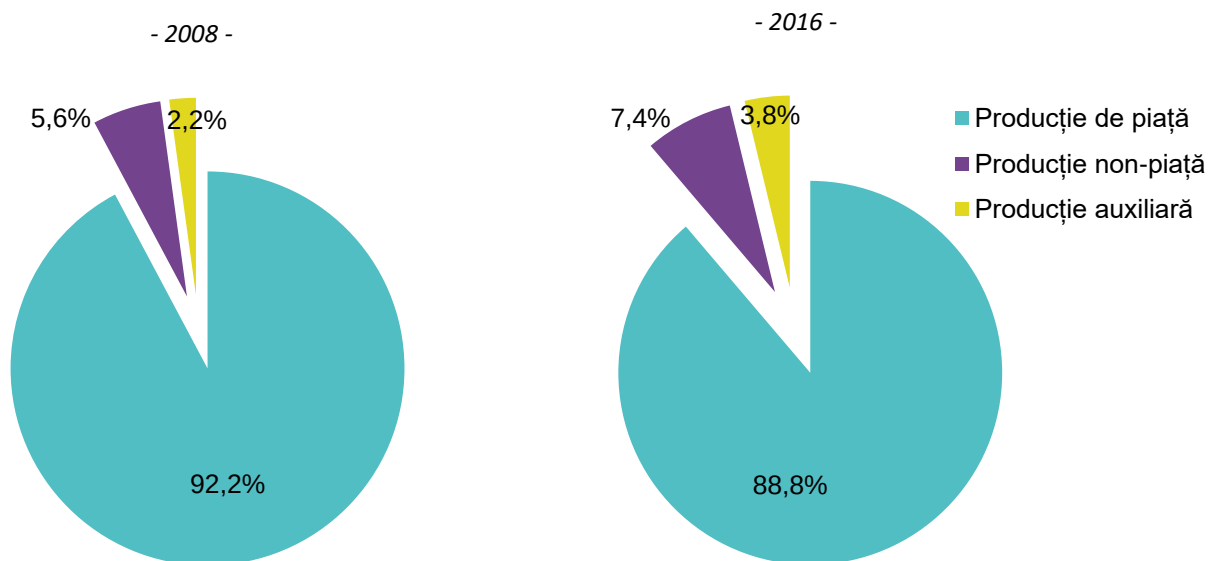
Graficul 3.11. Populația ocupată din EGSS pe tipuri de activități de mediu în anii 2008 și 2016
