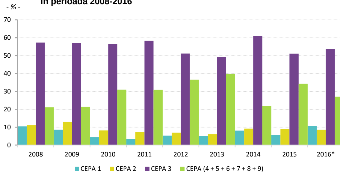
Graficul 4.3. Structura consumului intermediar pe principalele domenii de mediu CEPA în perioada 2008-2016
