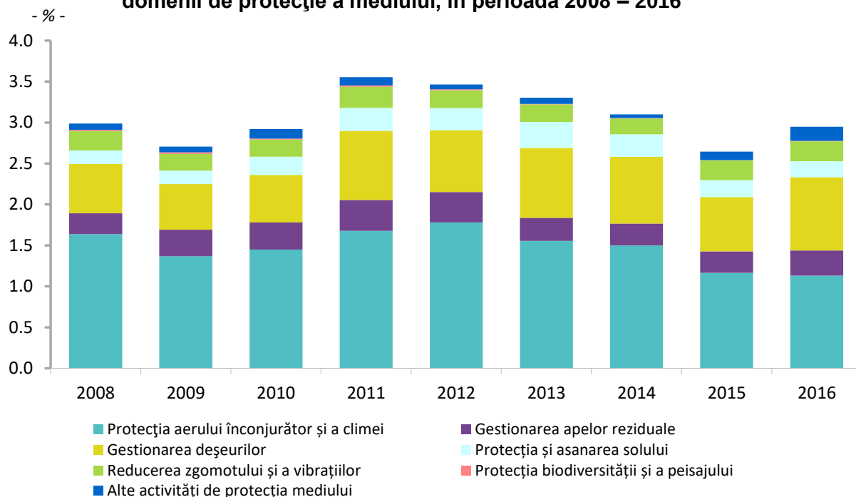
Graficul 3.2. Ponderea în PIB a valorii producției de bunuri și servicii de mediu, pe domenii de protecție a mediului, în perioada 2008 – 2016
