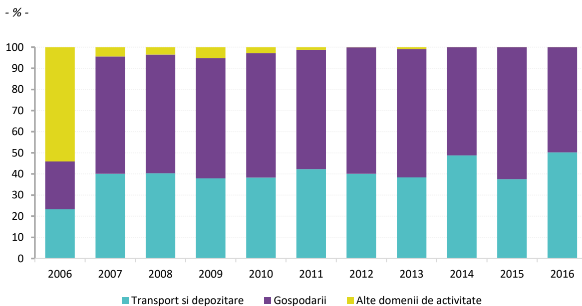
Graficul 5.9. Distribuția taxelor pe transport pe principalele domenii de activitate în perioada 2006 – 2016
