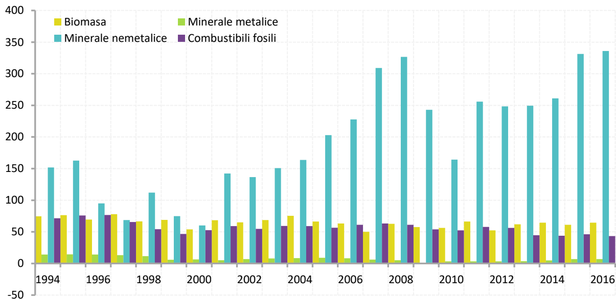
Graficul 1.6. Consumul intern de materiale pe principalele categorii, în perioada 1994 – 2016
