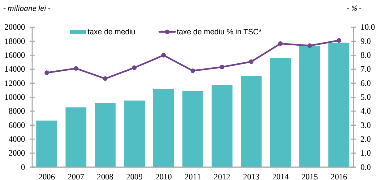
Graficul 5.2. Variația taxelor de mediu și a ponderii în TSC* în perioada 2006 – 2016
