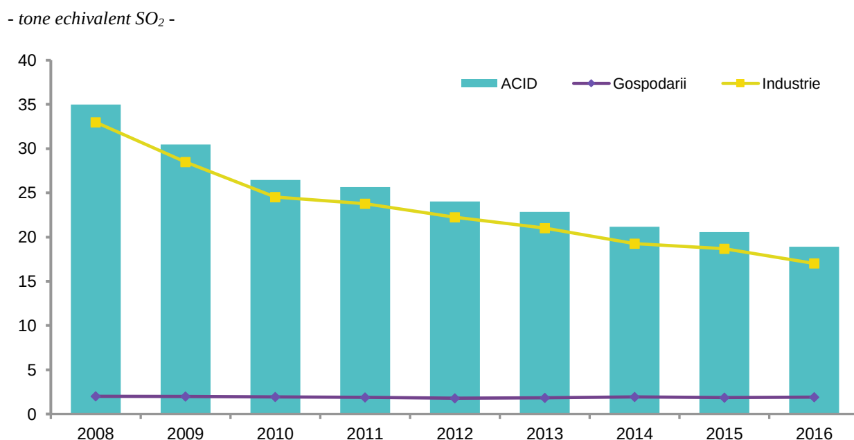
Graficul 2.9. Evoluția emisiilor compușilor acidifiante în industrie și gospodării în perioada 2008 – 2016
