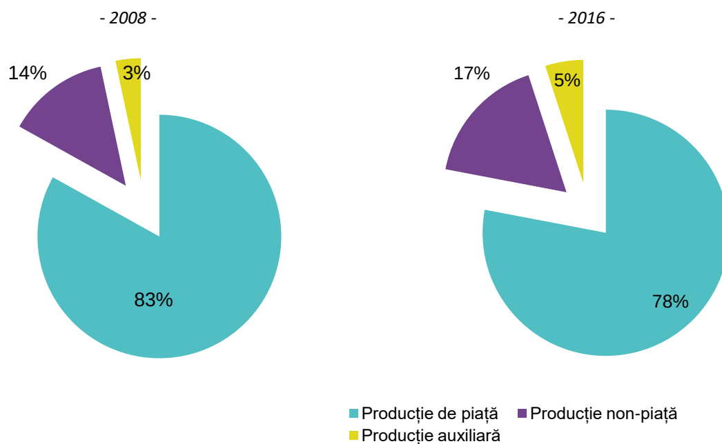
Graficul 3.9. Valoarea adăugată brută din EGSS pe categorii de activități rezultată în anii 2008 și 2016
