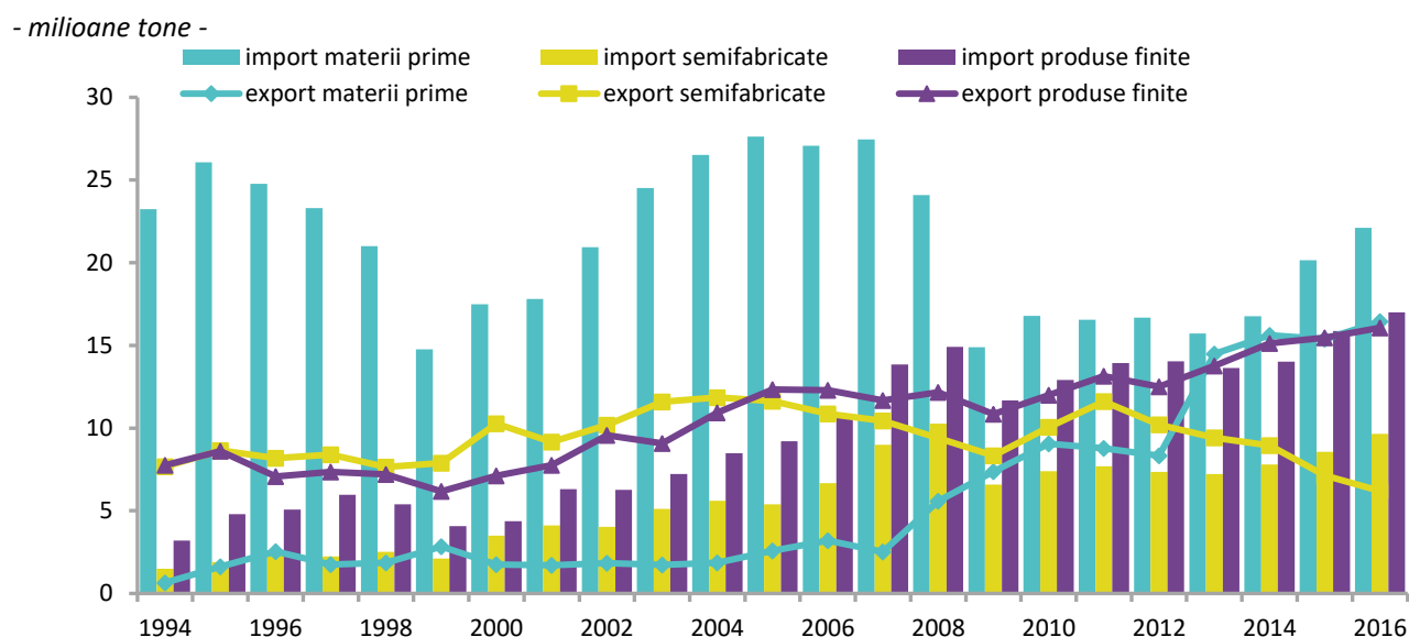
Graficul 1.11. Comerțul de materiale, pe stadii ale procesului de fabricație, în perioada 1994 – 2016
