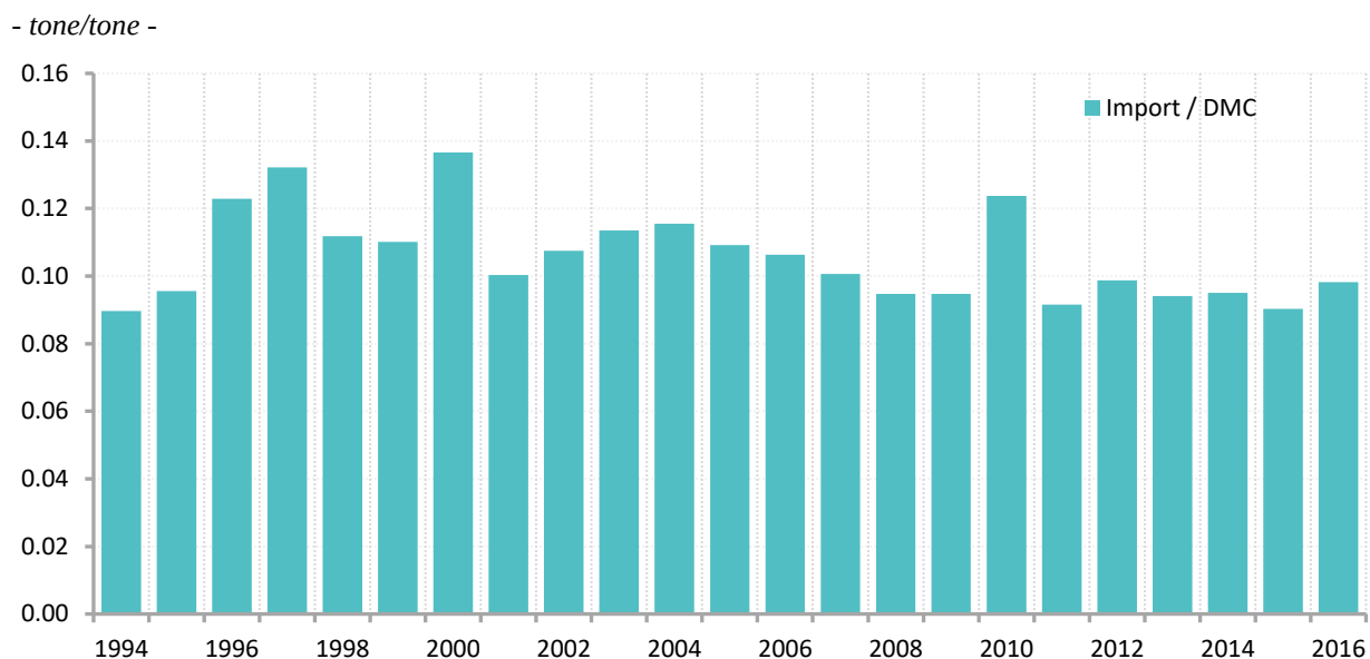
Graficul 1.17. Intensitatea comercială, în perioada 1994 – 2016
