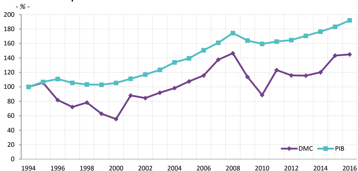
Graficul 1.12. Evoluția produsului intern brut și a consumului intern de materiale, în perioada 1994 – 2016
