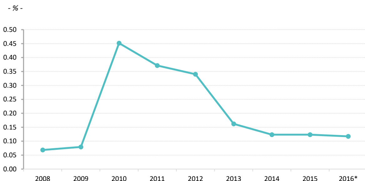
Graficul 4.9. Ponderea consumului final de servicii de protecția mediului al gospodăriilor populației în PIB în perioada 2008-2016
