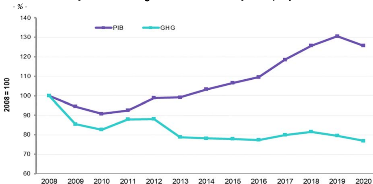
Graficul 2.5. Evoluția emisiilor de gaze cu efect de seră și a PIB, în perioada 2008-2020
