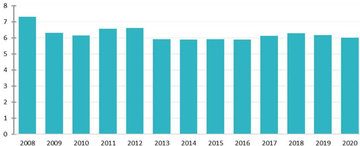
Graficul 2.7. Emisiile de gaze cu efect de seră pe locuitor în perioada 2008 – 2020
