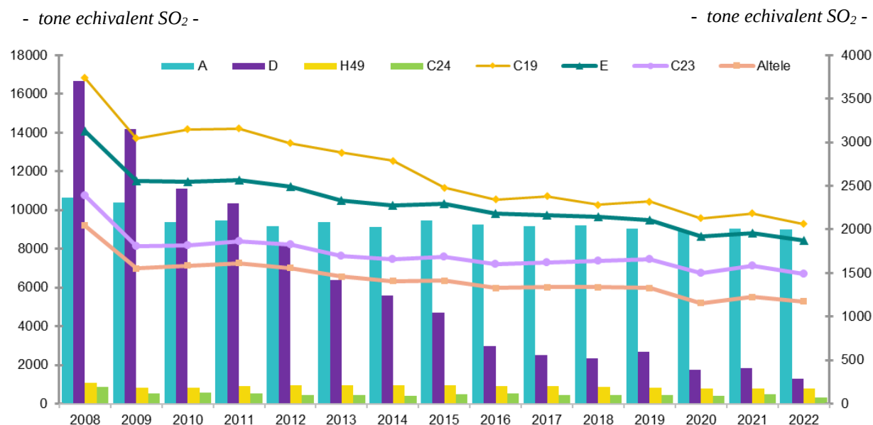
Graficul 2.8. Evoluția emisiilor de gaze acidifiante pe principalele activități economice în perioada 2008 – 2022
