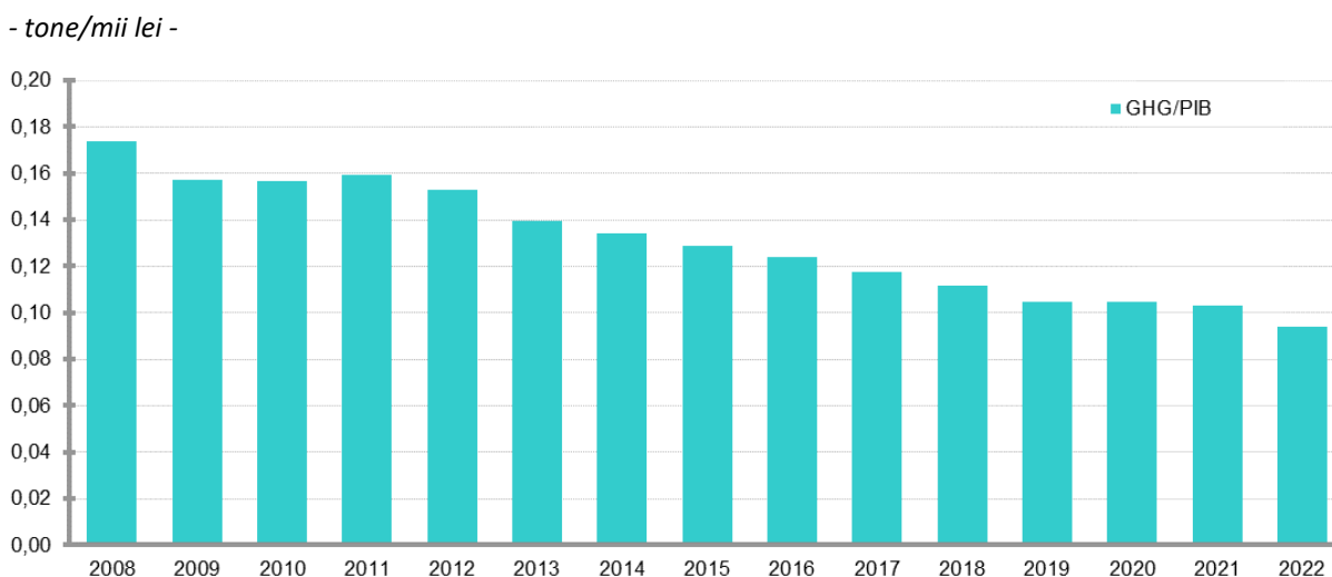
Graficul 2.6. Evoluția intensității emisiilor de gaze cu efect de seră, în perioada 2008-2022
