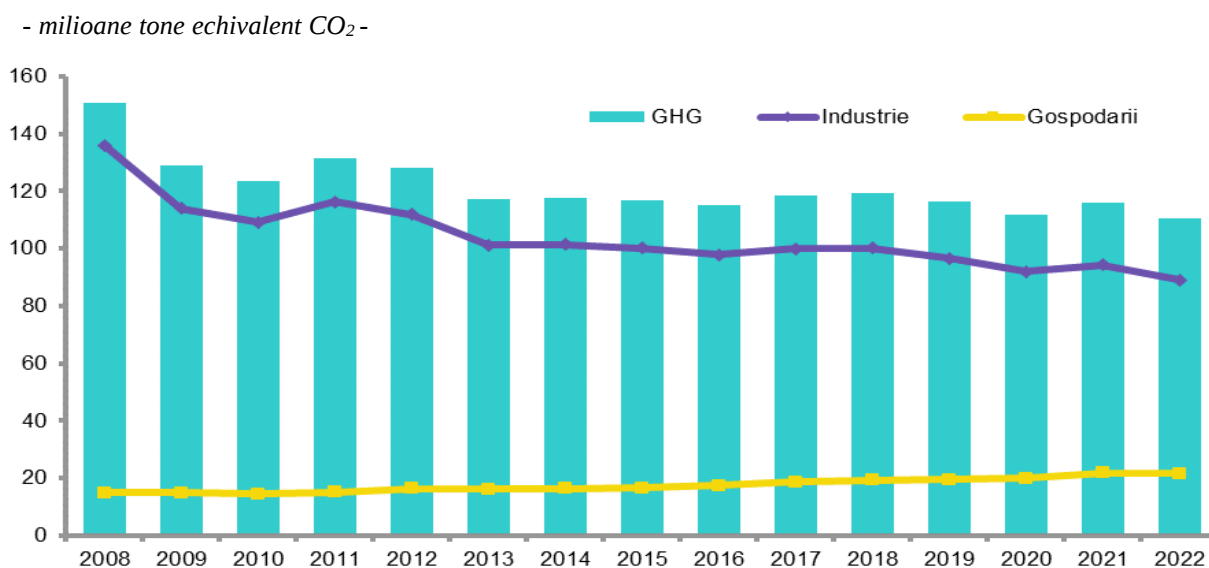
Graficul 2.1. Evoluția emisiilor gazelor cu efect de seră din industrie și gospodării, în perioada 2008 – 2022
