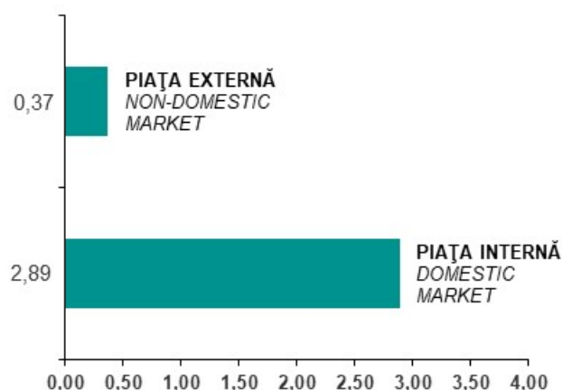
Contribuția pe cele două piețe (internă și externă) la evoluția IPPi în luna noiembrie 2024 comparativ cu luna octombrie 2024 Contribution to IPPi evolution, by markets (domestic and non-domestic) in November 2024 in comparison with the October 2024
