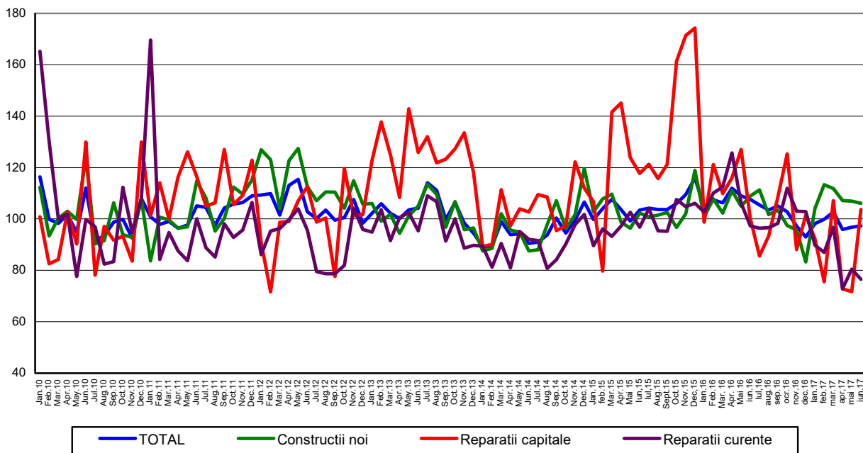
Evoluția lunară a lucrărilor de construcții, pe elemente de structură, conform CAEN Rev. 2 - ianuarie 2010 – iunie 2017- (serie ajustată în funcție de numărul de zile lucrătoare și de sezonabilitate)
