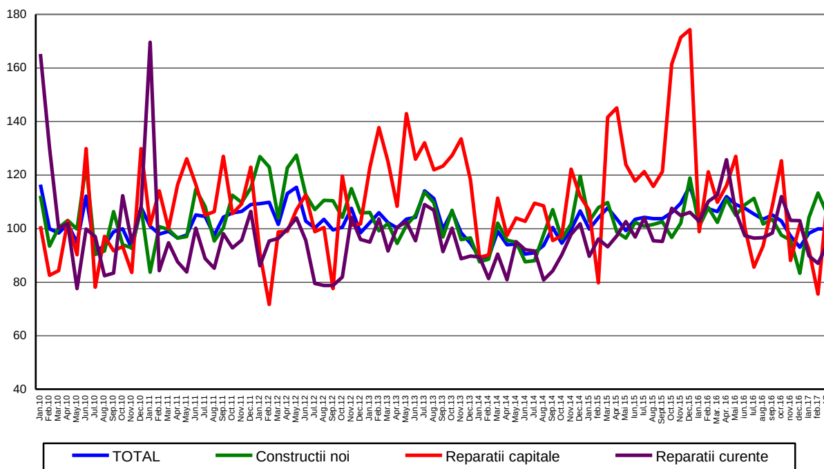
Evoluția lunară a lucrărilor de construcții, pe elemente de structură, conform CAEN Rev. 2 - ianuarie 2010 – martie 2017- (serie ajustată în funcție de numărul de zile lucrătoare și de sezonabilitate)
