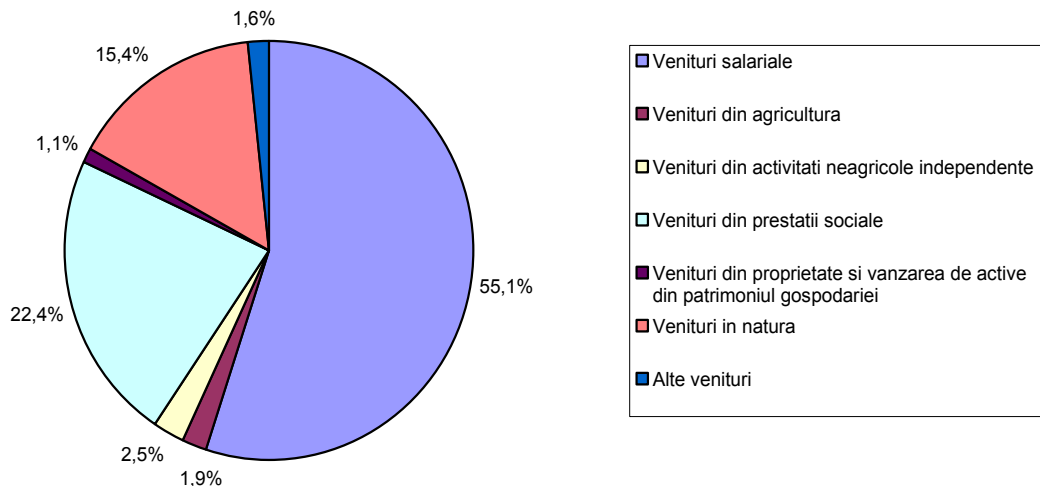
Structura veniturilor totale ale gospodariilor, pe surse de formare, în trimestrul I 2016
