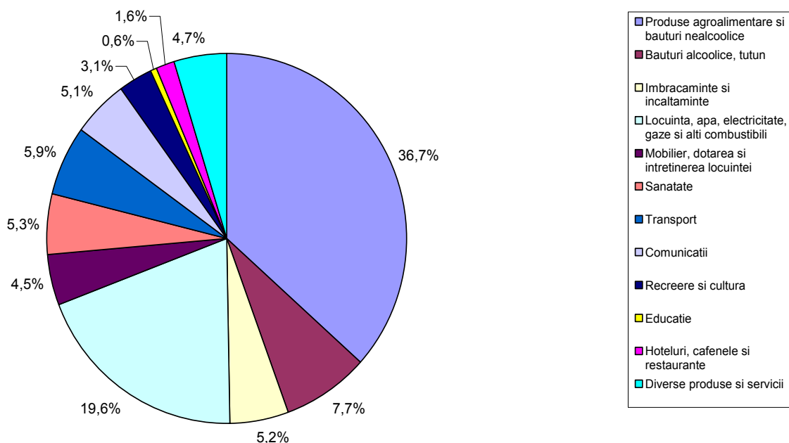
Structura cheltuielilor totale de consum pe destinații, în trimestrul I 2016
